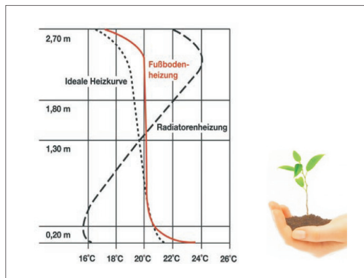
2 - Temperaturprofile der verschiedenen Heizsysteme
