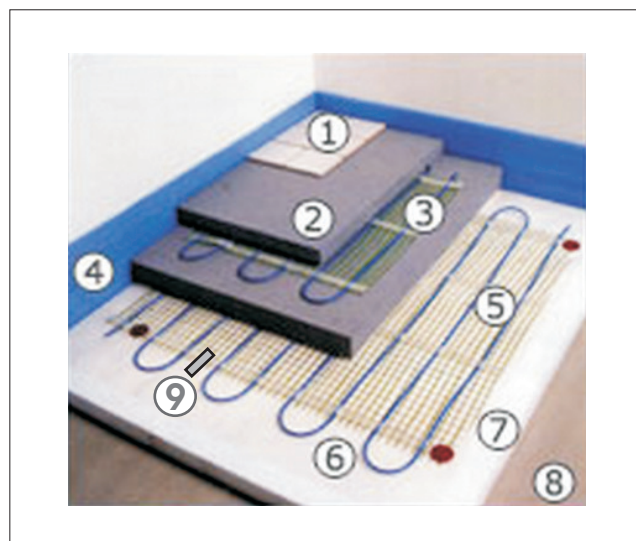
1 - Technischer Aufbau einer Elektro-Fußbodenspeicherheizung
